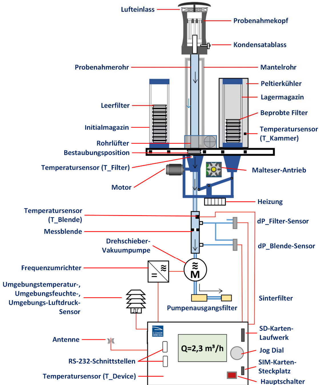
Abbildung 4: Schematischer Aufbau PNS T-DM
