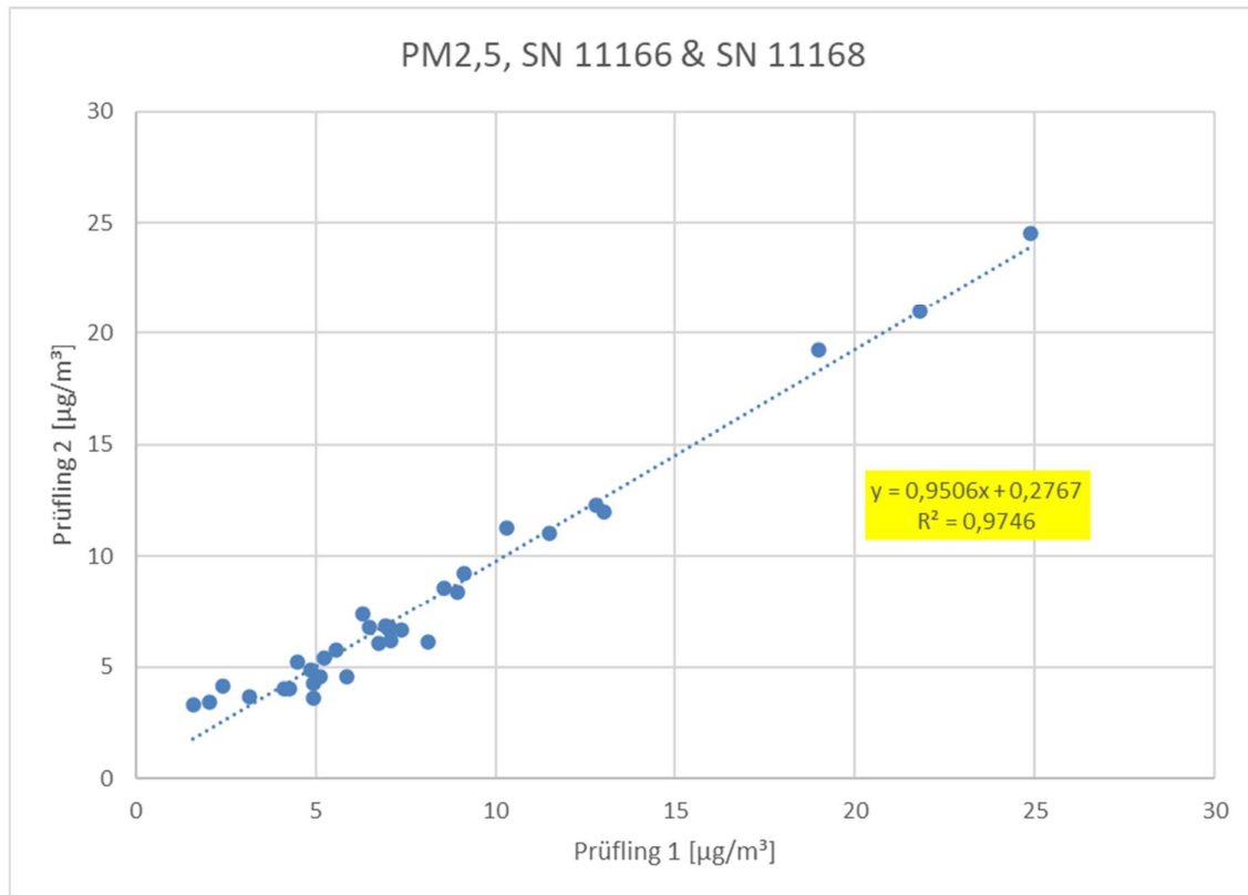
Abbildung 27: SN 11166 vs. SN 11168, PM 2,5
