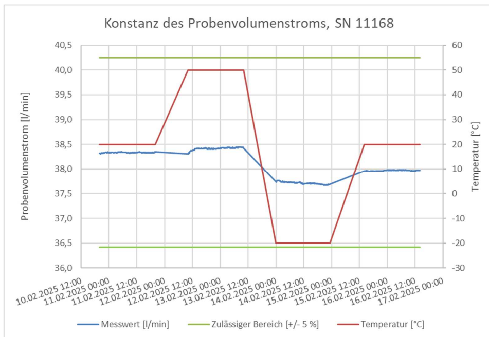
Abbildung 22: Verlauf des Proben­volumenstroms, PNS T-DM-3.1, SN 11168
