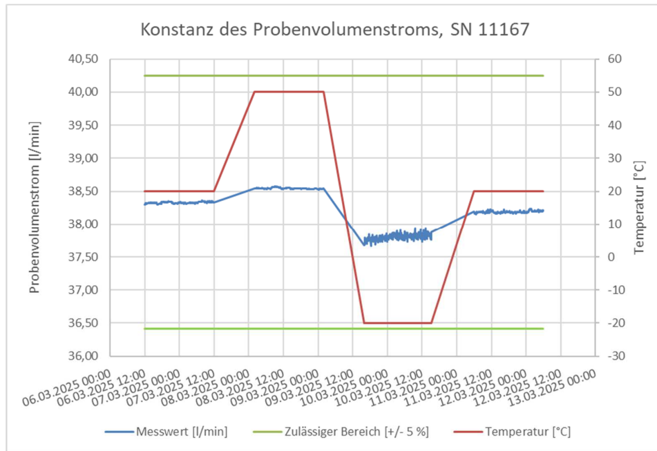
Abbildung 23: Verlauf des Probenvolumenstroms, PNS T-DM-6.1, SN 11167
