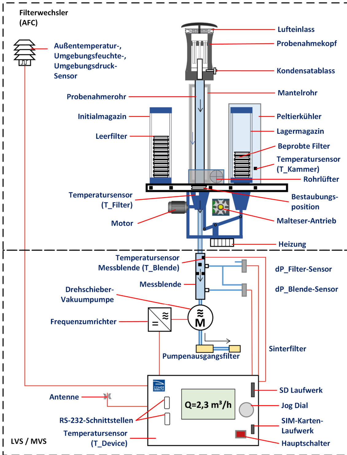
Abbildung 6: Schematischer Aufbau PNS DM (=LVS/MVS + AFC-DM)
