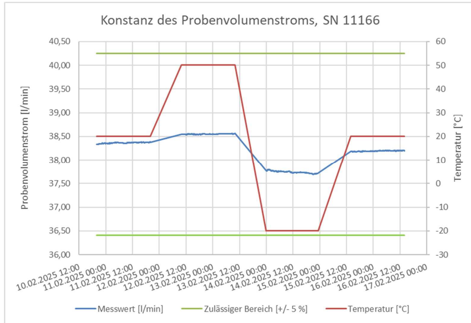
Abbildung 21: Verlauf des Proben­volumenstroms, PNS T-DM-3.1, SN 11166
