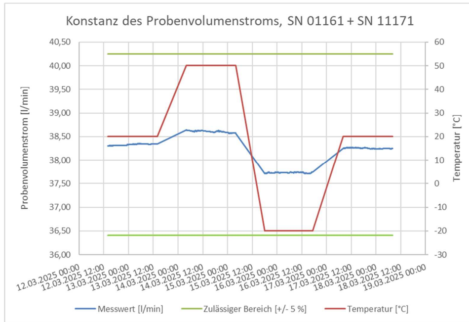
Abbildung 25: Verlauf des Probenvolumenstroms, PNS DM-3.1, SN 01161+SN 11171
