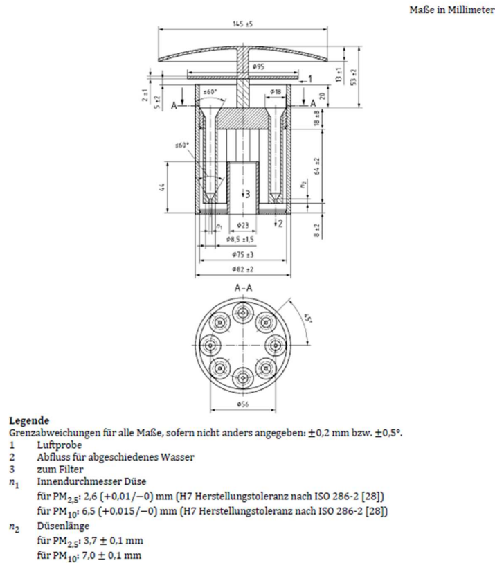
Abbildung 12: Schematischer Aufbau des Probeneinlasses gemäß Anhang A der DIN EN 12341
