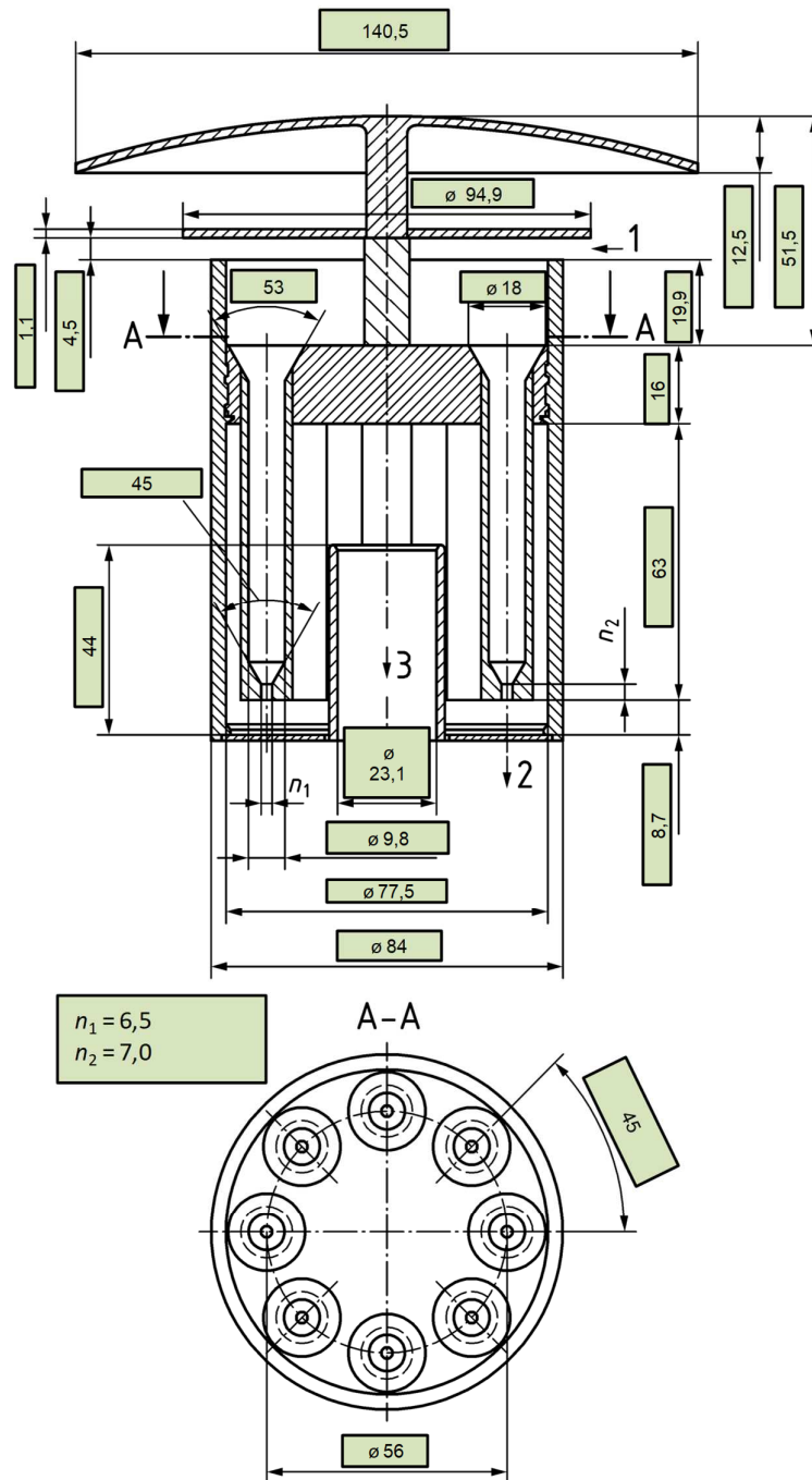
Abbildung 18: Standard-Probeneinlass für PM 10 , Ist-Maße
