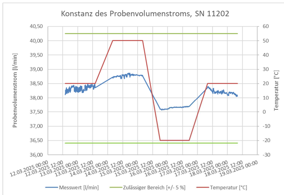
Abbildung 24: Verlauf des Probenvolumenstroms, PNS DMC-6.1, SN 11202
