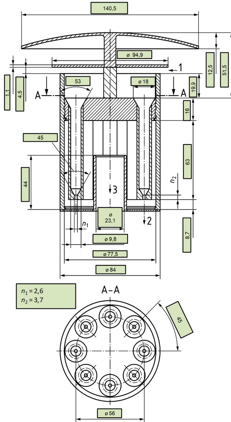
Abbildung 15: Standard-Probeneinlass für PM 2,5 , Ist-Maße
