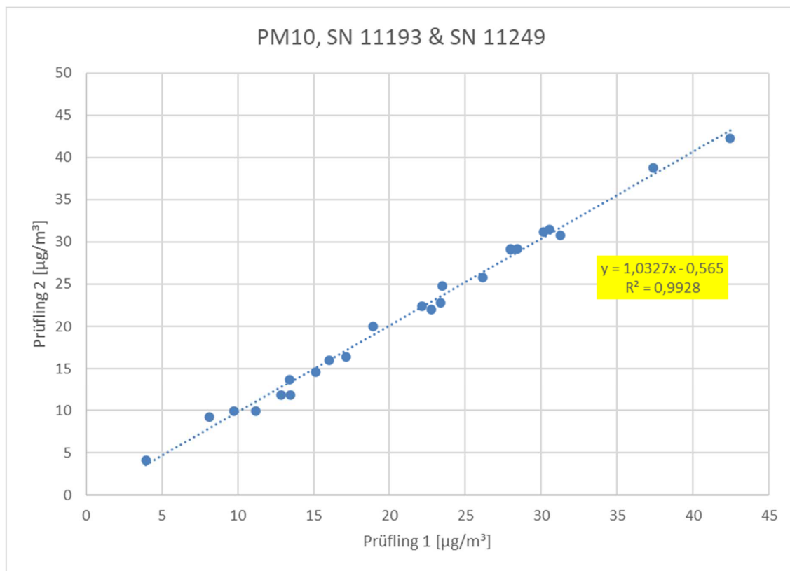
Abbildung 28: SN 11193 vs. SN 11249, PM 10
