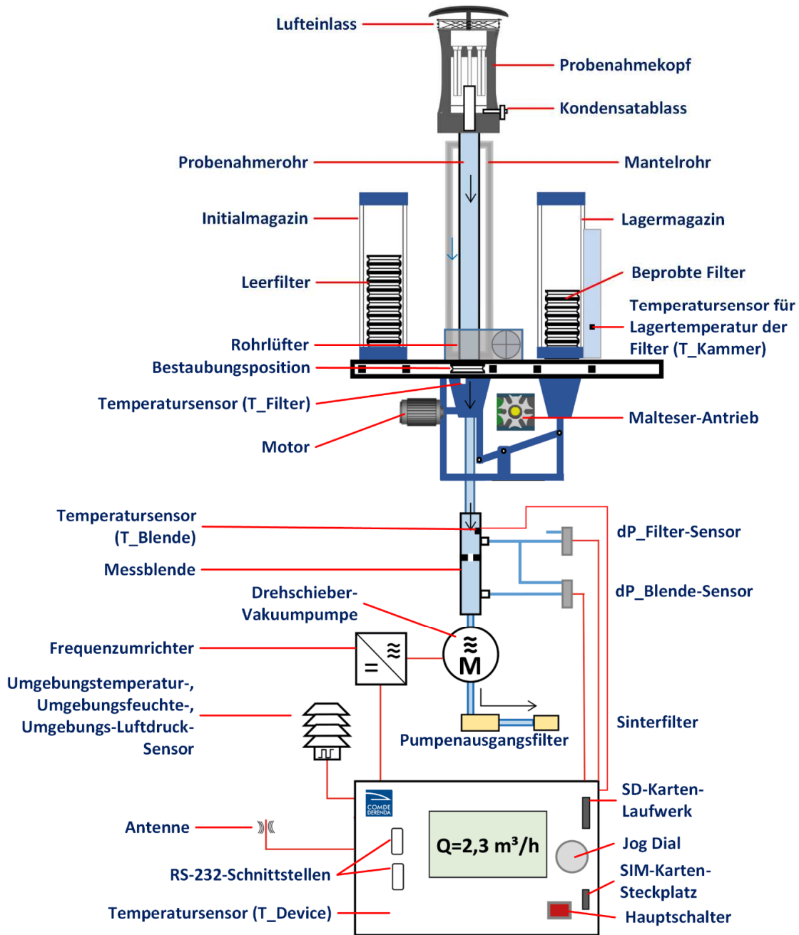
Abbildung 5: Schematischer Aufbau PNS DMC
